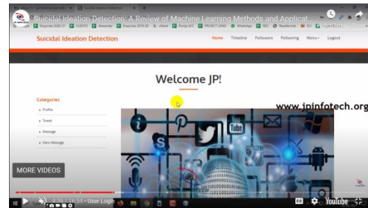
Fig.4. Welcome page.
